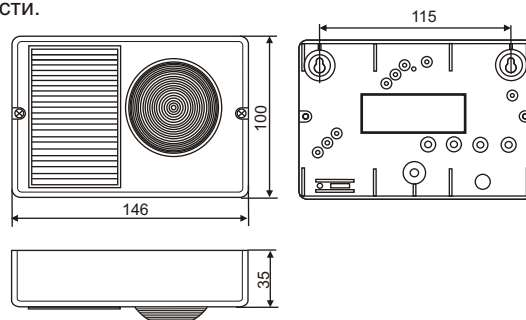
Рис.1. Габаритные и установочные размеры.
