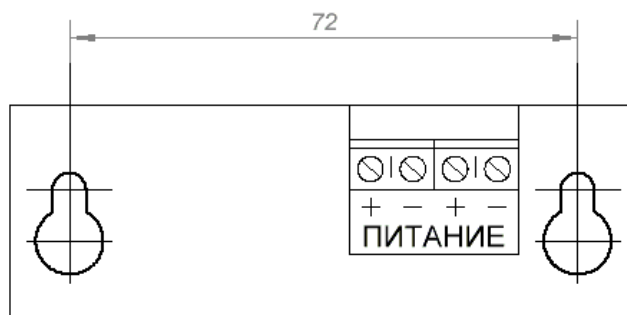
Рис.1 Схема подключения и установочные размеры оповещателя
