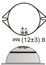
Рис.2 Схема подключения и диаграмма направленности оповещателя.
